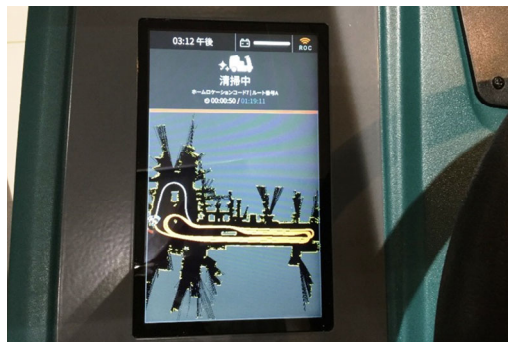
事前の手動運転で簡単ルート設定
