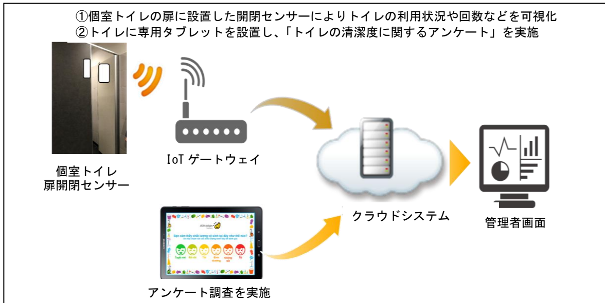
「トイレ IoT サービス」概要図
